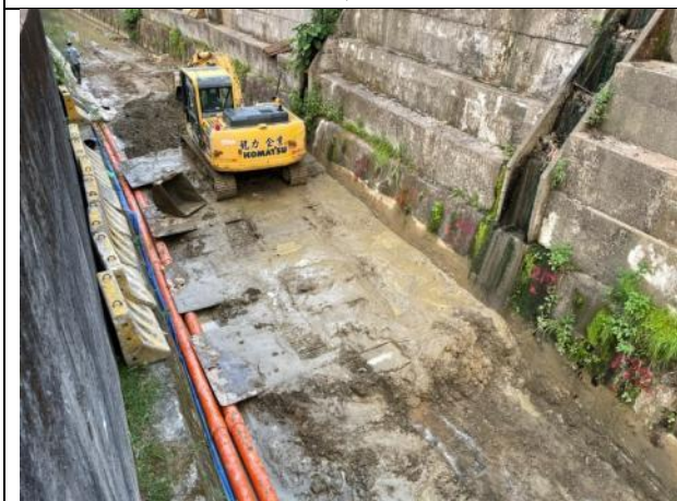
臨時引流管 設置日期 110/9/19
