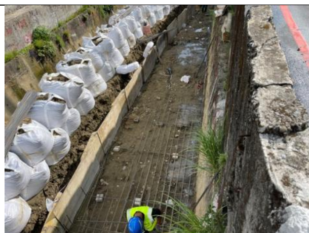
太空包圍堰堵水 設置日期 110/11/3
