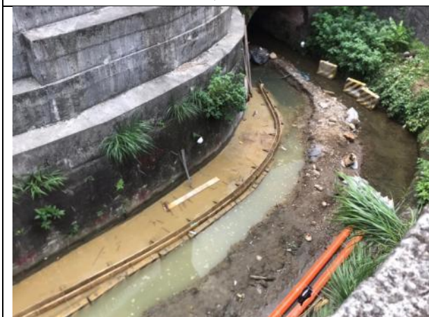
臨時引流管 設置日期 110/9/17
